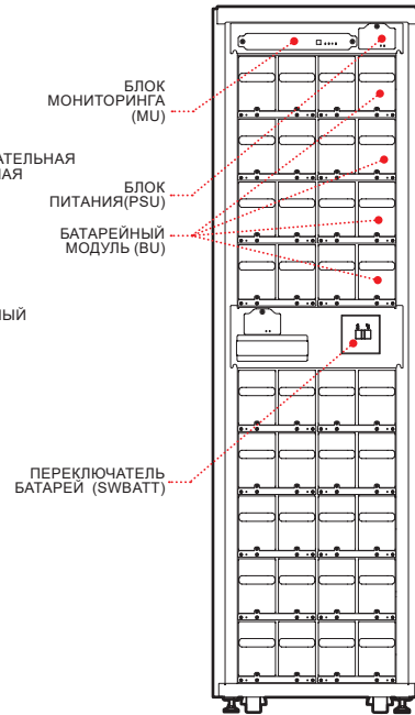
ВТС 170 MPW Батарейный шкаф (лицевая сторона)
